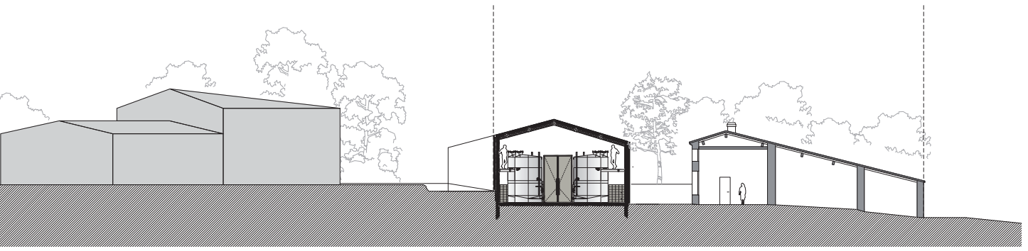
COUPE TRANSVERSALE
